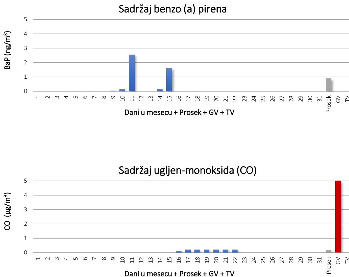
Grafikon 2: Dnevne vrednosti sadržaja benzo (a) pirena i ugljenmonoksida na mernom mestu Bulevar Veljka Vlahovića u toku avgusta 2023. godine
